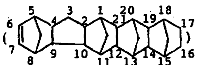
Nonacyclo[11.11.15.8.113.20.115.18.02.10.04.9 012.21.014.19]-eicos-6-ene
