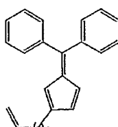
2-(but-3-enyl)-6,6-diphenylpentafulvene
