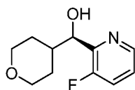
Enantiomer a1
