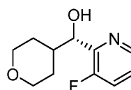
Enantiomer b1
