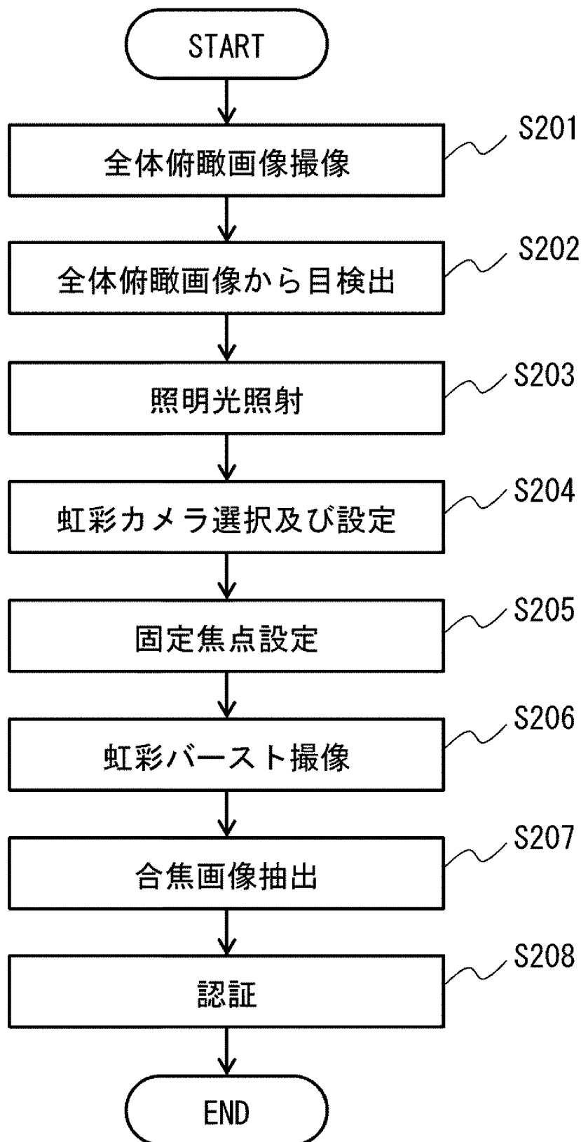
[図5] <ウォークスルー認証処理>
