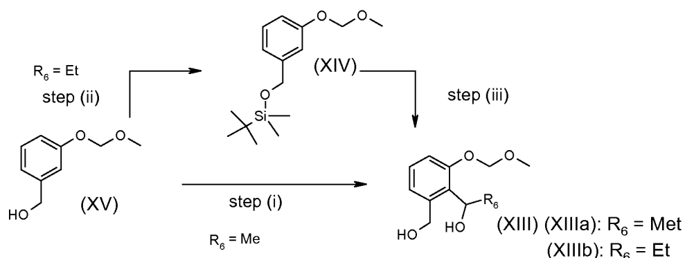
Scheme 8a
