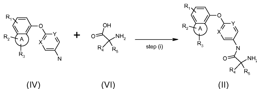
Scheme 2a
