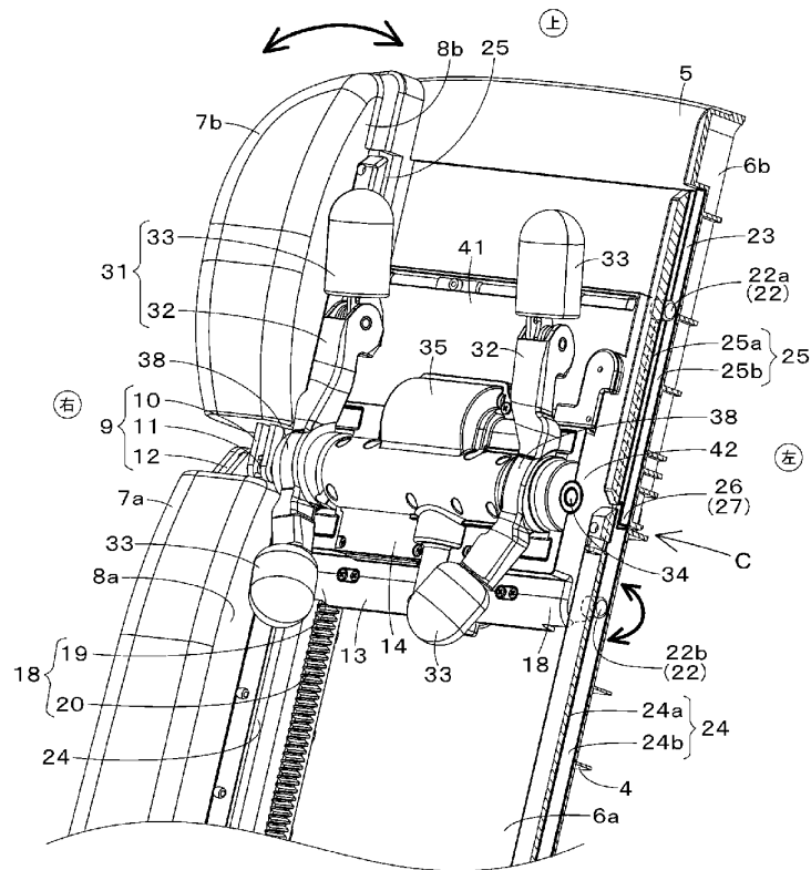
A-A断面
