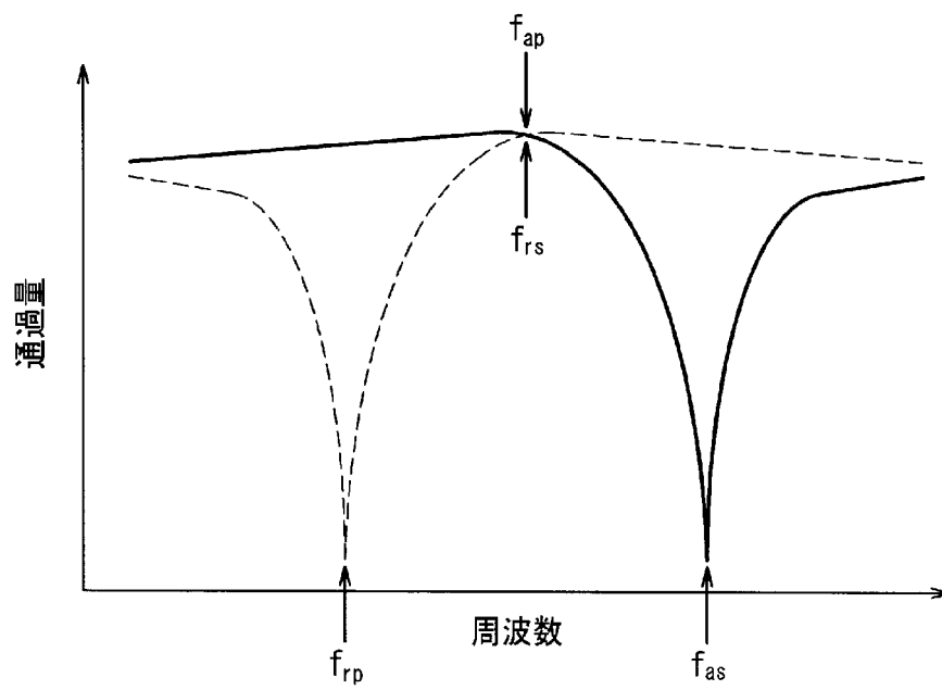
共振器の周波数特性
