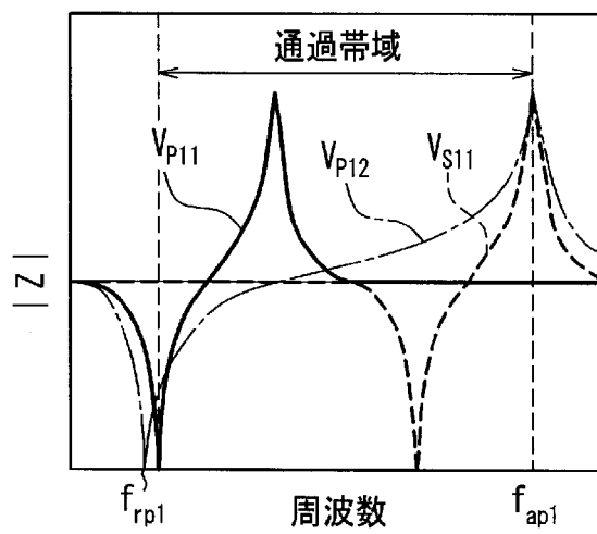
各共振器の周波数特性
