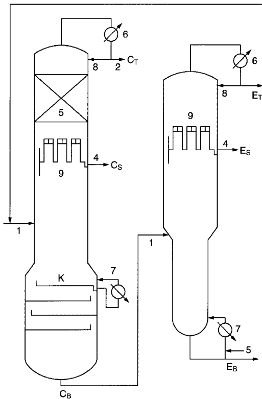
AA... 連続多段蒸留塔C
