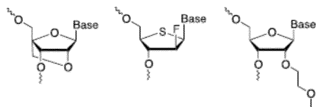
LNA
