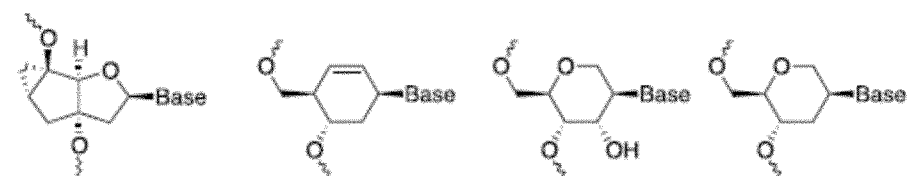
tc-DNA
