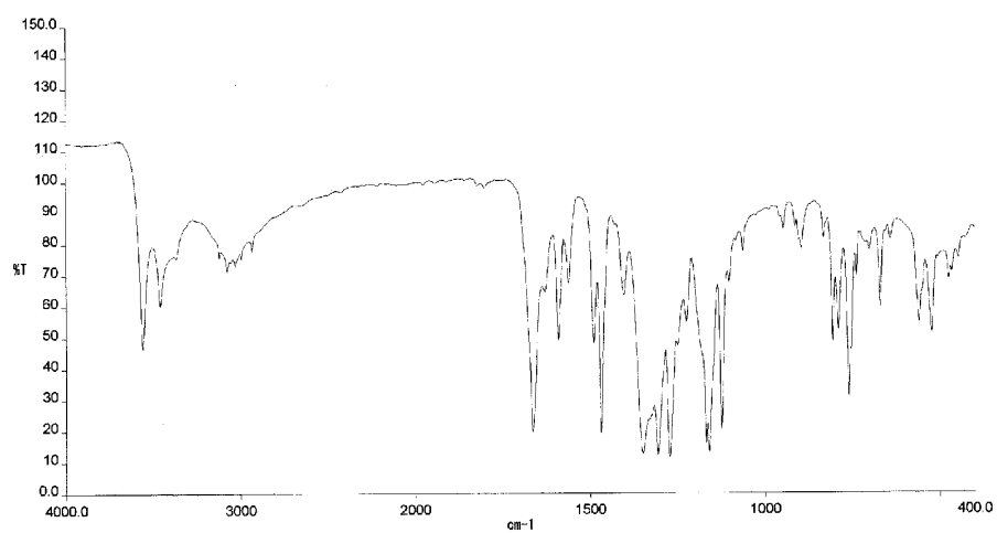
水和物の赤外線吸収スペクトル（I R）
