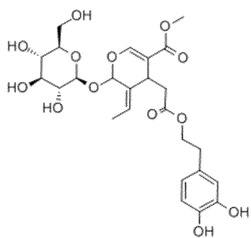
(B) Oleuropein
