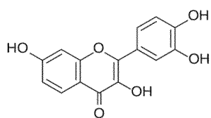
(A) Fisetin
