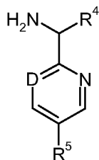
Formula (D)
