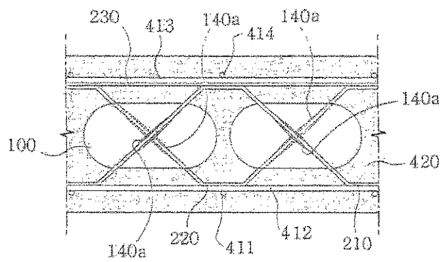
A-A Section
