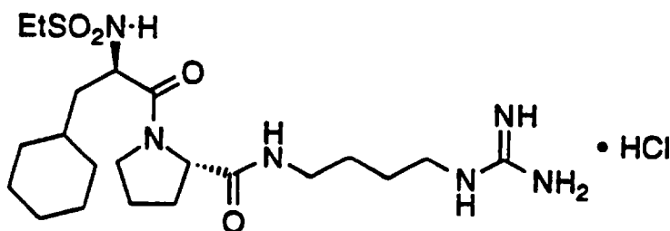
EtSO 2 -D-Cha-Pro-Agm·HCl
