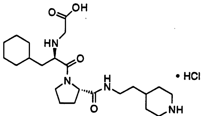
HO 2 CCH 2 -D-Cha-Pro-4-NHCH 2 CH 2 -piperidine·HCl
