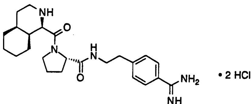
D-1-Piq-Pro-p-NHCH 2 CH 2 -C 6 H 4 C(=NH)NH 2 ·2HCl
