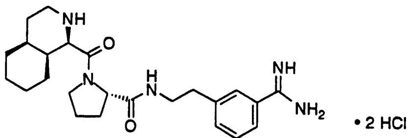
D-1-Piq-Pro-m-NHCH 2 CH 2 -C 6 H 4 C(=NH)NH 2 ·2HCl
