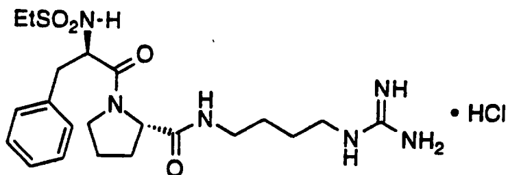
EtSO 2 -D-Phe-Pro-Agm·HCl
