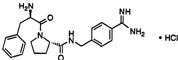
D-Phe-Pro-p-NHCH 2 CH 2 C 6 H 4 C(NH)NH 2 ·HCl
