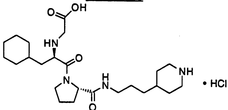
HO 2 CCH 2 -D-Cha-Pro-4-NHCH 2 CH 2 CH 2 -piperidine·HCl
