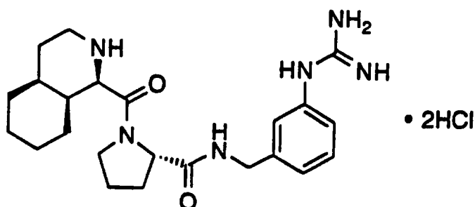
D-1-Piq-Pro-m-NHCH 2 C 6 H 4 NHC(NH)NH 2 · 2HCl
