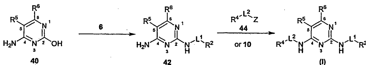
Scheme (IV)
