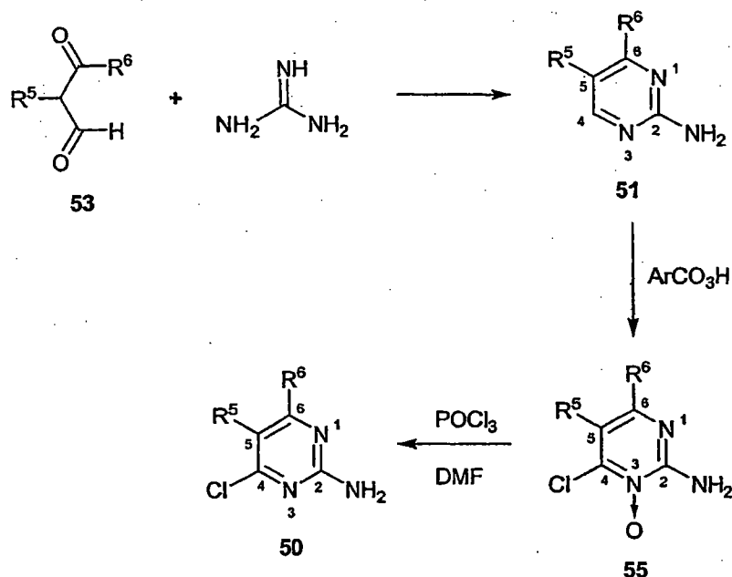
Scheme (Va)
