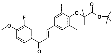
1-(4-Methoxy-3-fluorophenyl)-3-(4-carboxydimethylmethoxy-3,5-dimethylphenyl)prop-2-en-1-one :
