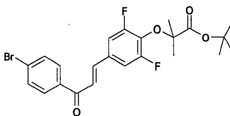
1-(4-Bromophenyl)-3-(4-tert-butyloxycarbonyldimethylmethoxy-3,5-difluorophenyl)prop-2-en-1-one :
