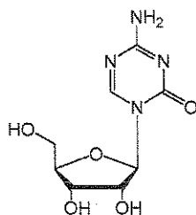
5-Azacytidine.
