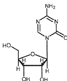
5-Azacytidine.
