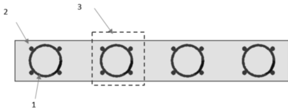
用螺旋钢筋加强的结构墙的俯视图
