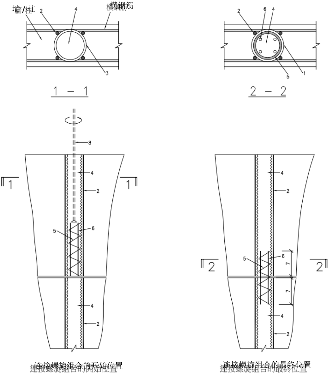
一种以螺旋钢筋组合连接加固墙和柱的方案
