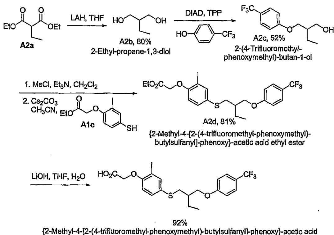
Scheme A2
