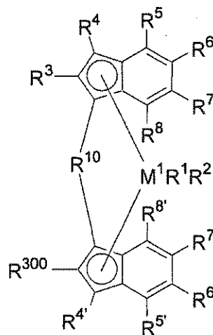
meso/pseudomeso isomer
