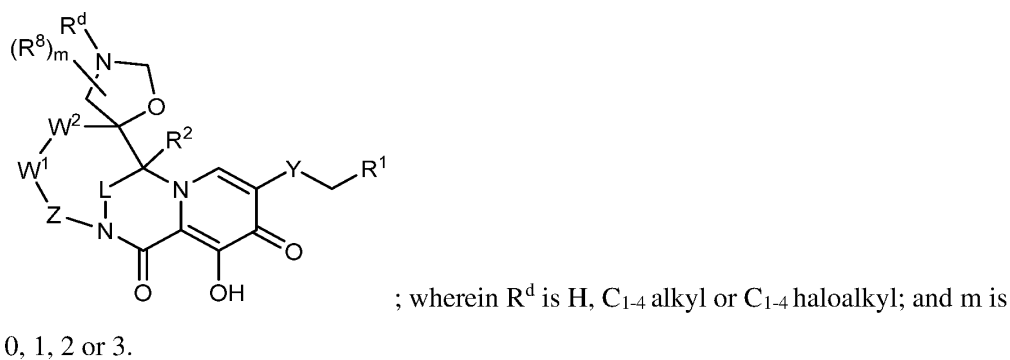
I-D
