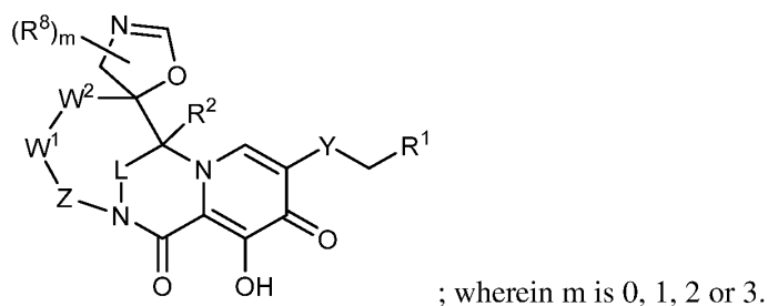
I-B
