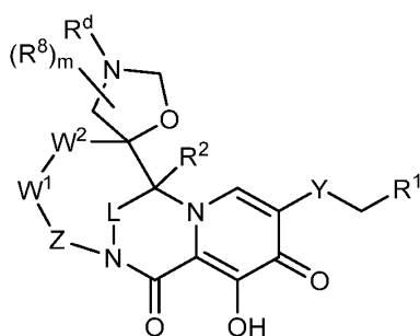
I-D
