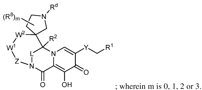
I-C
