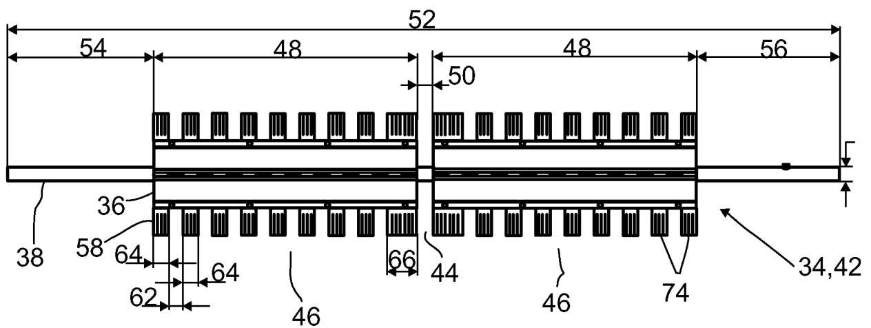
FIG.3 A-A
