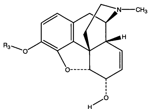
(Ia),
