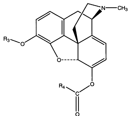
(IIIa).
