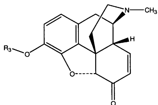
(IIa),
