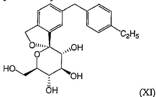
[Formula 15]
