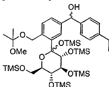
[Formula 26]
