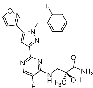
Formula IC
