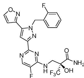
Formula IC
