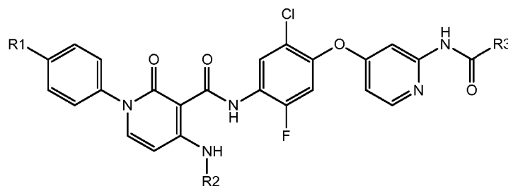
Formula Ih.4
