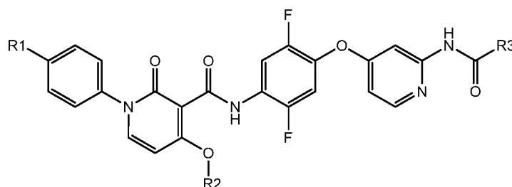
Formula Ic
