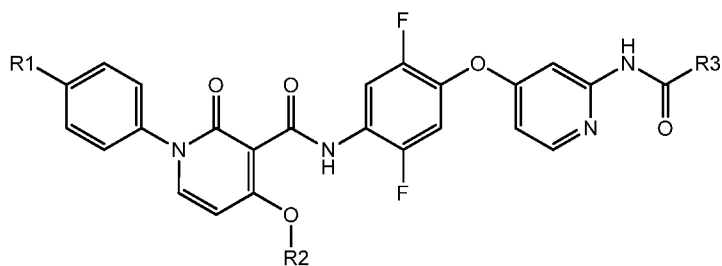
Formula Ic
