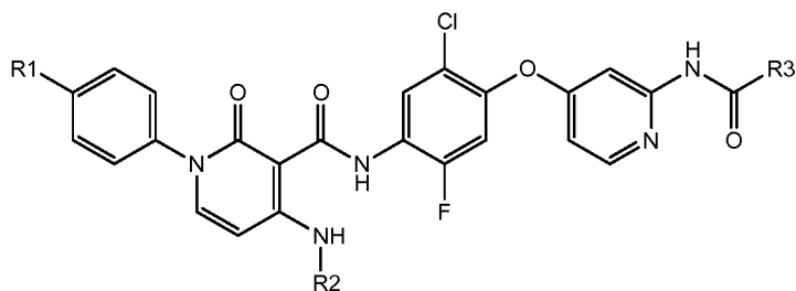
Formula Ih.1
