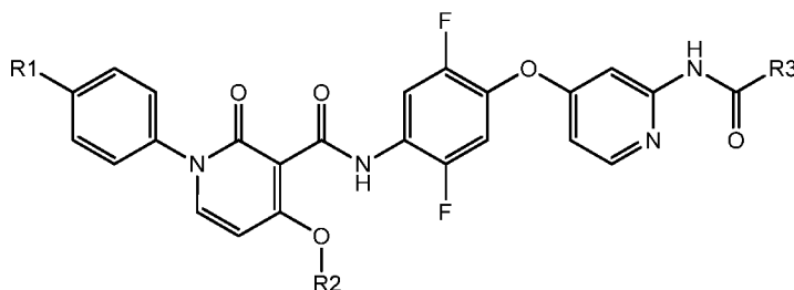
Formula Ic
