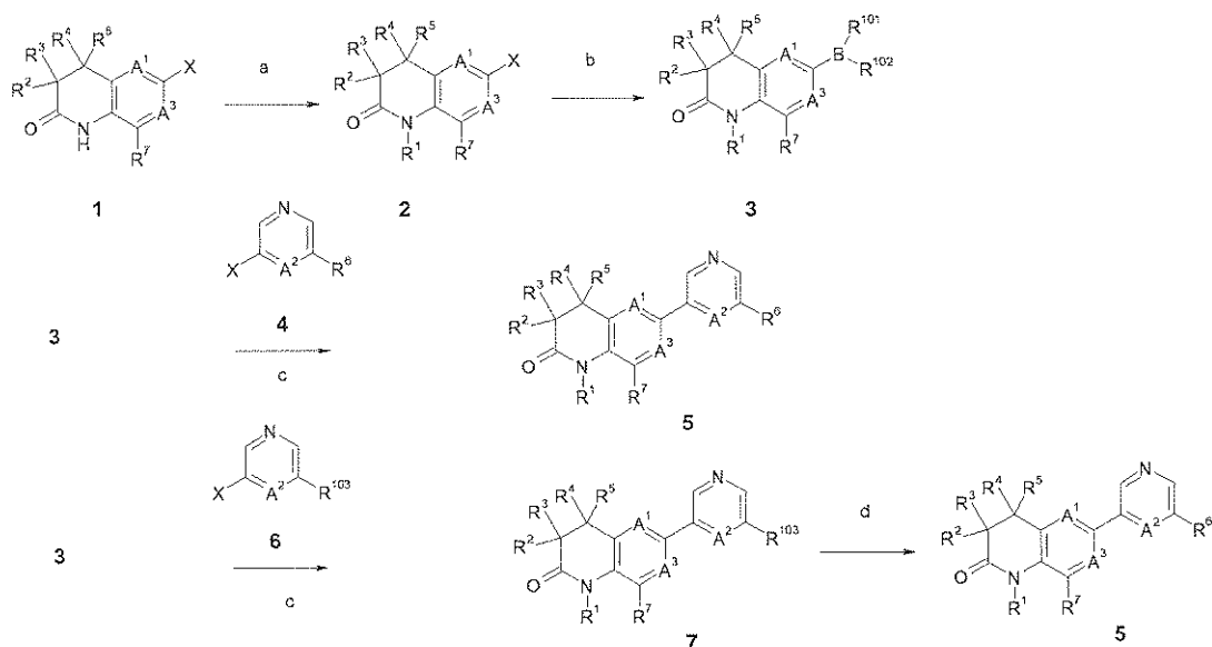
Scheme 1a
