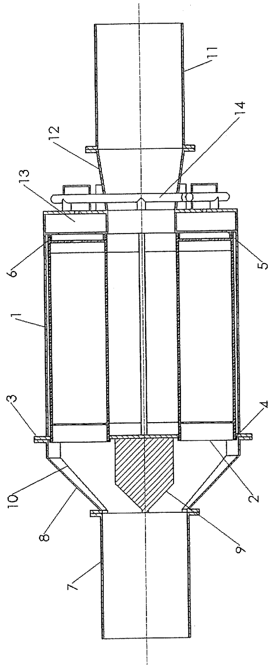
SECTION A-A
