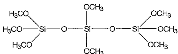
Octamethoxytrisiloxane (OMOTS)
