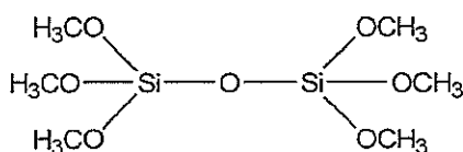
Hexamethoxydisiloxane (HMODS)
