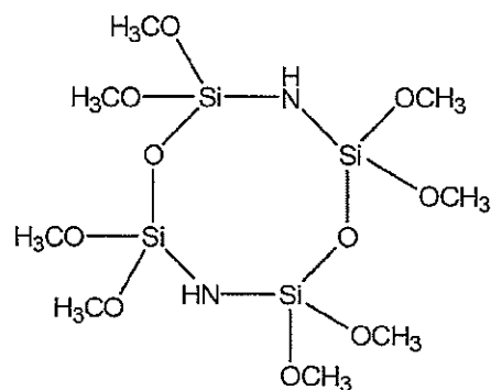
Octamethoxycyclicsilazoxane (OMCS)
