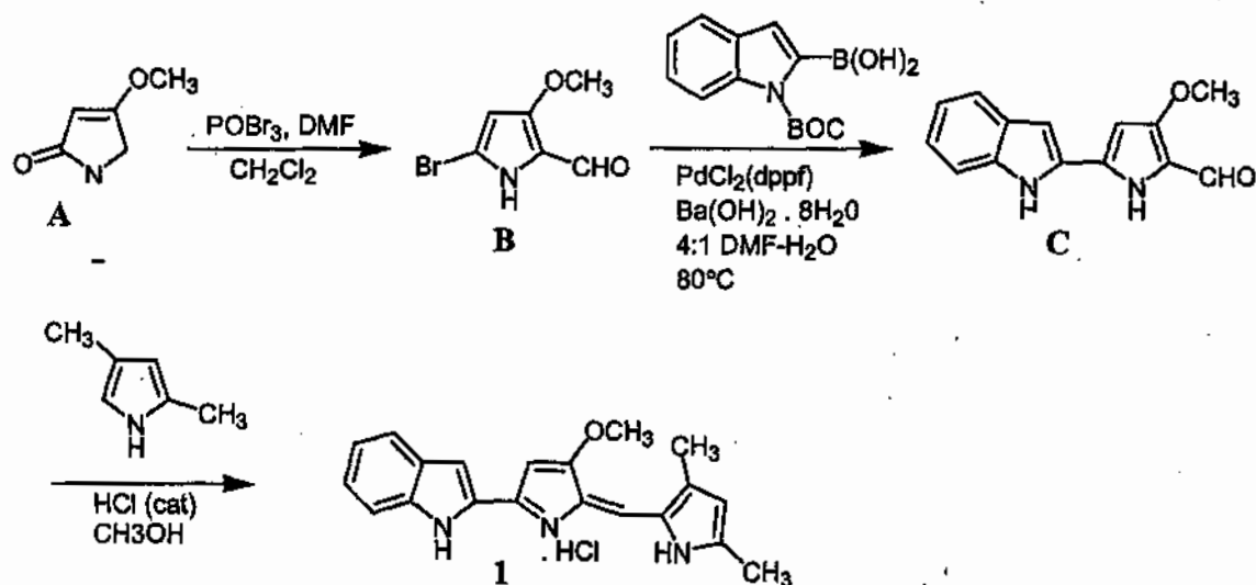
Scheme 2a
