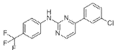
VAF347
