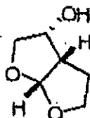
(3R,3aS,6aR)-hexahydrofuro[2,3-b]furan-3-ol
