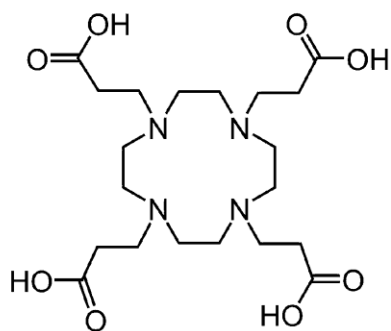
DOTPA
