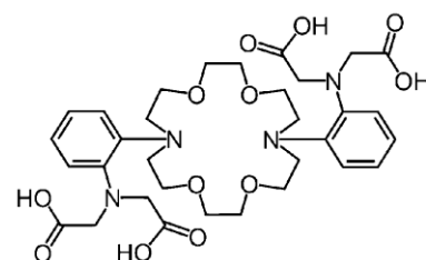
macropid
