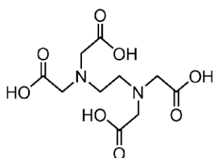
EDTA
