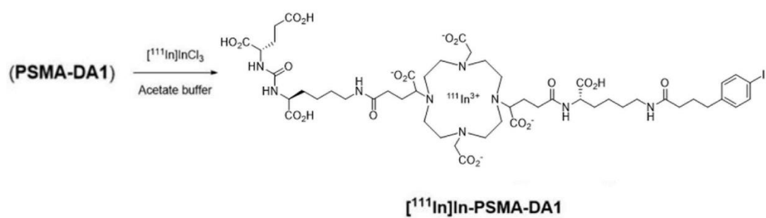
Scheme(V-2)
