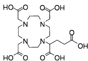
DOTAGA
