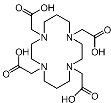
TETA
