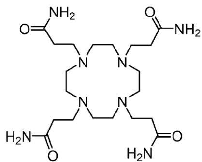
DOTAM
