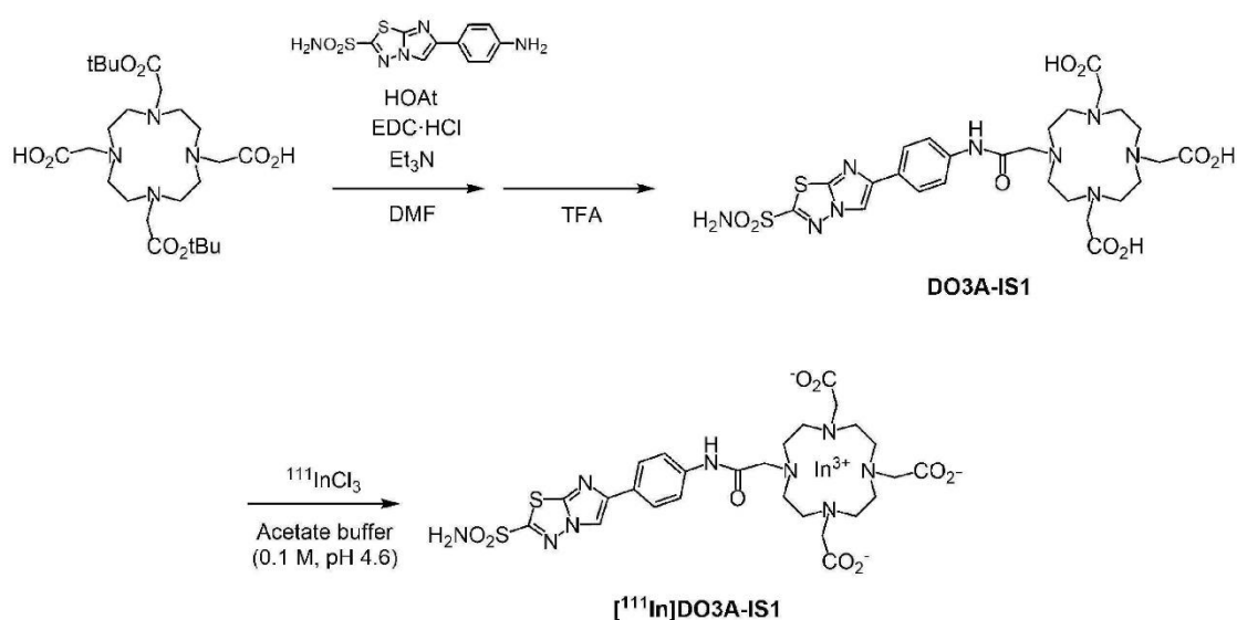
Scheme(IV)
