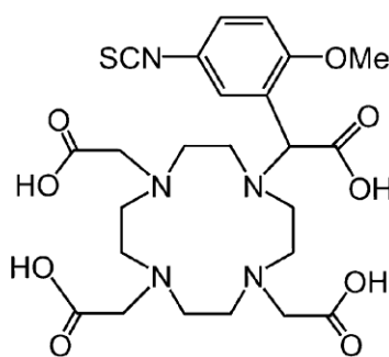
MeO-DOTA-NCS
