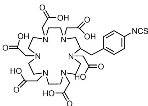
HEHA-NCS
