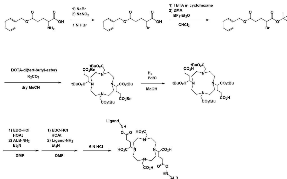
Scheme(II)
