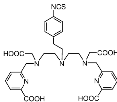
p-SCN-Bn-H 4 neunpa
