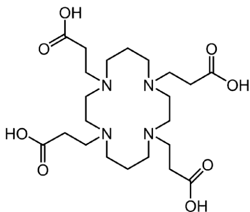
TETPA
