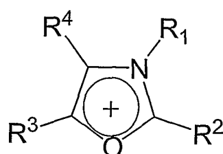
Oxazolium
