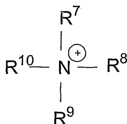
Ammonium
