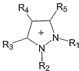
Pyrazolium
