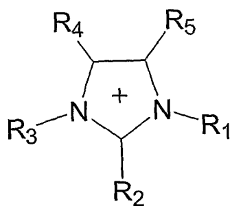
Imidazolium
