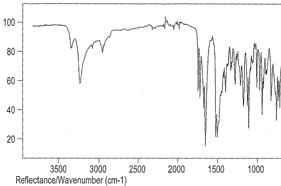
FIG. 11A
