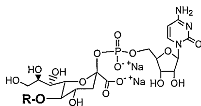
CMP-KDN-5-O-R
