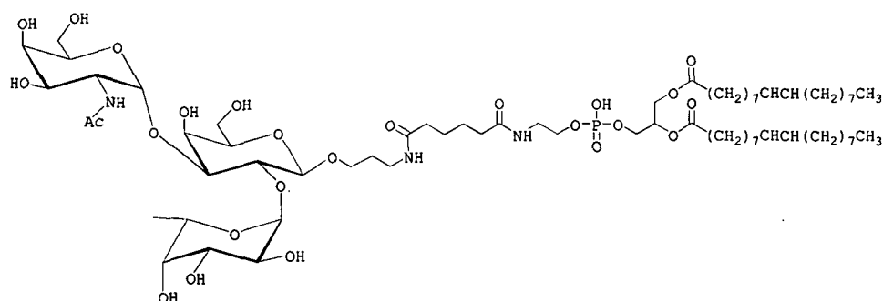
FSL-A
