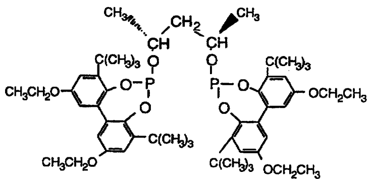
Ligand K
