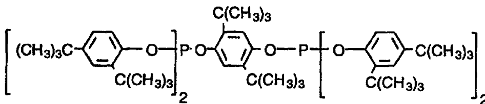
Ligand T
