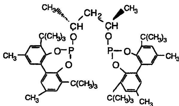
Ligand J
