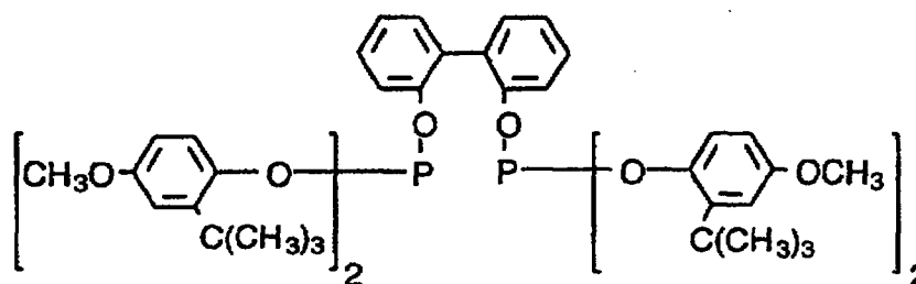
Ligand V
