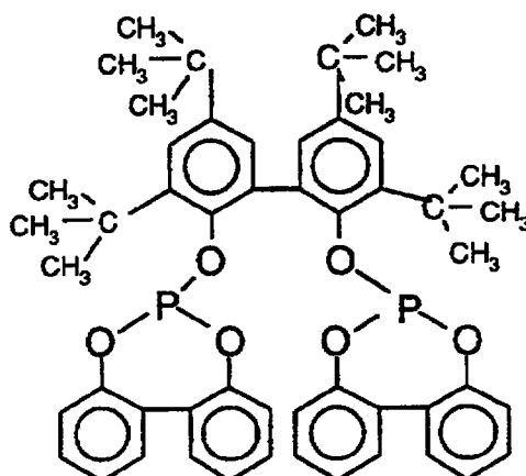
Ligand F
