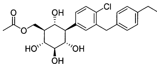
((1 S ,2 R ,3 R ,4 S ,5 R ,6 R )-3-(4-chloro-3-(4-ethylbenzyl)phenyl)-2,4,5,6-tetrahydroxycyclohexyl)methyl acetate
