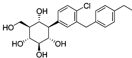
5 (R = Et)
