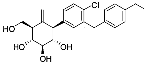
(1 R ,2 R ,3 S ,4 S ,6 R )-4-(4-chloro-3-(4-ethylbenzyl)phenyl)-6-(hydroxymethyl)-5-methylenecyclohexane-1,2,3-triol
