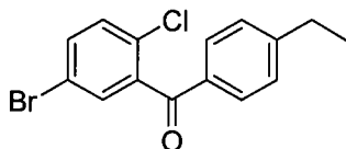
7 (R = Et)
