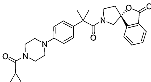
(1R)-1'-(2-{4-[4-(Cyclopropylcarbonyl)piperazin-1-yl]phenyl}-2-methylpropanoyl)-3H-spiro[2-benzofuran-1,3'-pyrrolidin]-3-one
