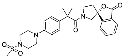
(1R)-1'-(2-Methyl-2-{4-[4-(methylsulfonyl)piperazin-1-yl]phenyl}propanoyl)-3H-spiro[2-benzofuran-1,3'-pyrrolidin]-3-one
