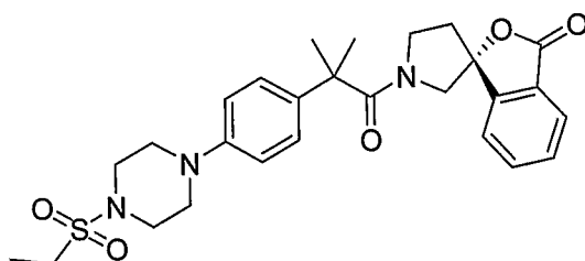
(1R)-1'-(2-{4-[4-(ethylsulfonyl)piperazin-1-yl]phenyl}-2-methylpropanoyl)-3H-spiro[2-benzofuran-1,3'-pyrrolidin]-3-one
