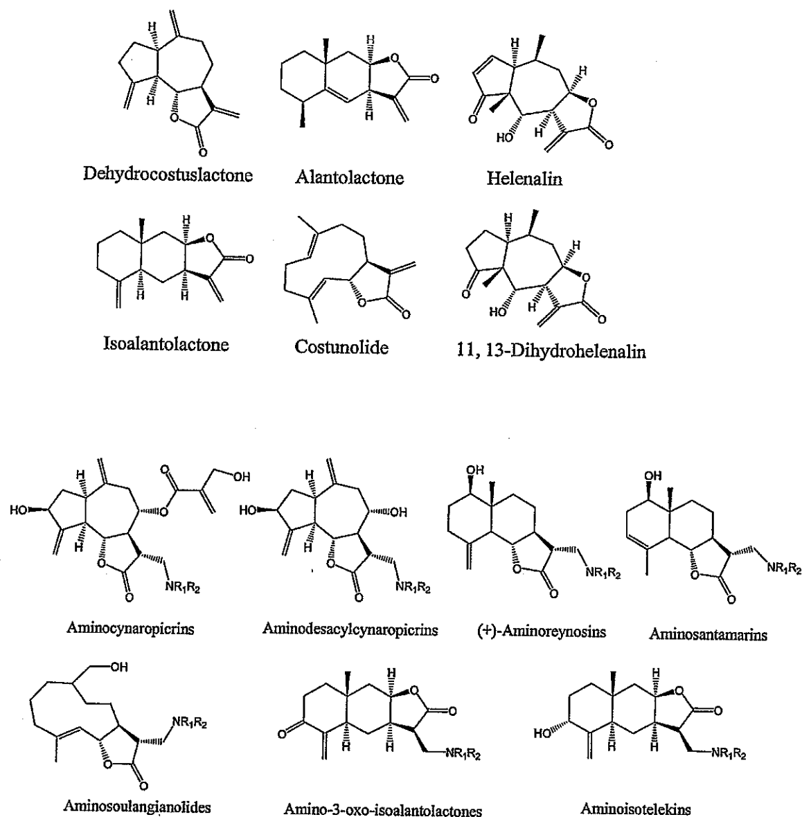
Scheme VI
