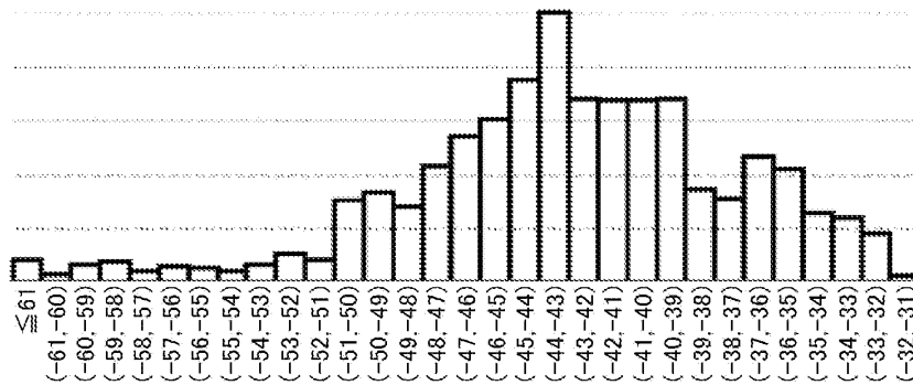
一定距離での単一受信機の受信電波強度ヒストグラム
