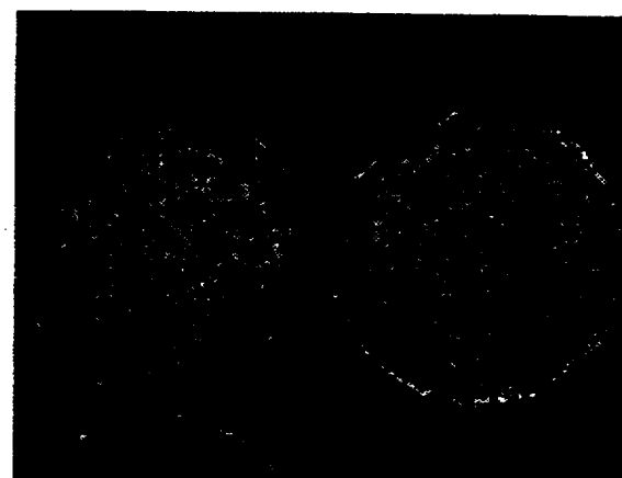
(400 Si)
