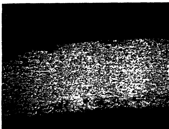
(100 YN + 400 Si)
