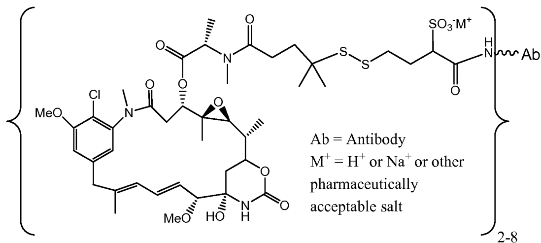
Ab-sulfo-SPDB-DM4
