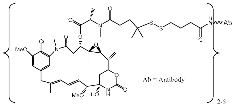
Ab-SPDB-DM1
