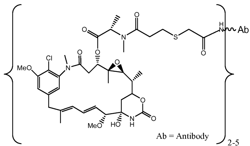
Ab-SIA-DM1
