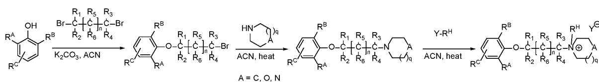
Scheme A:
