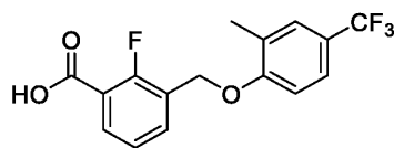
1-101
