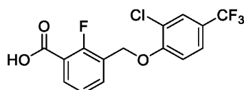
1-55
