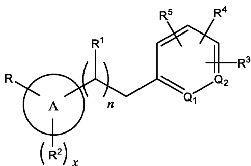
(XVIII)
