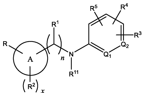
(XVII)
