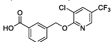
35-1
