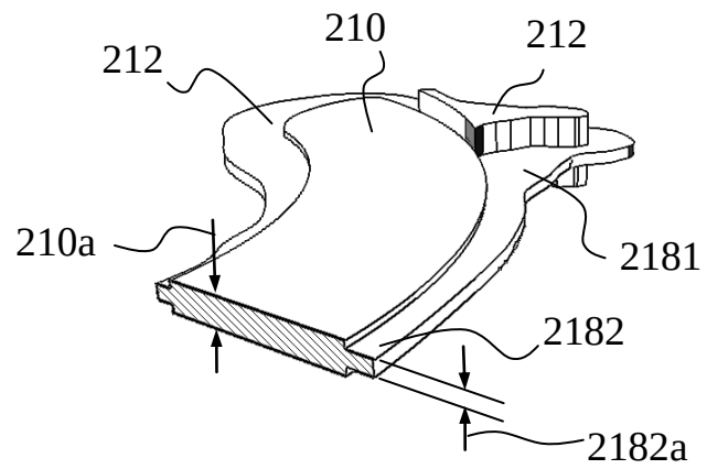
FIG. 5 (B-B)
