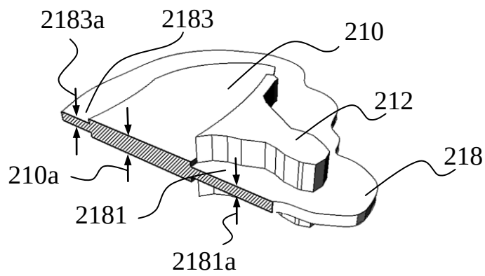
FIG. 4 (A-A)
