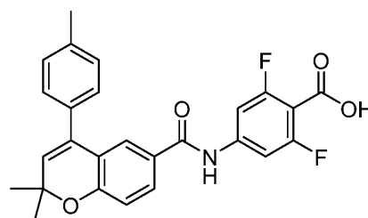
AGN 194574
