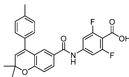
AGN 194574
