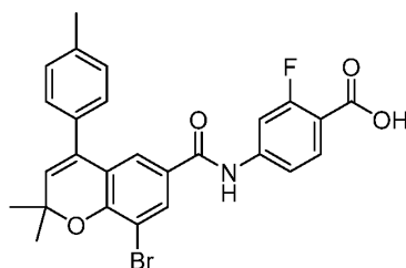
AGN 194301
