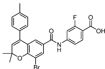
AGN 194301
