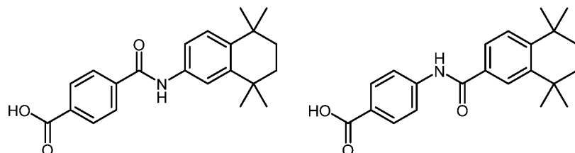
Tamibarotene (AM80)
