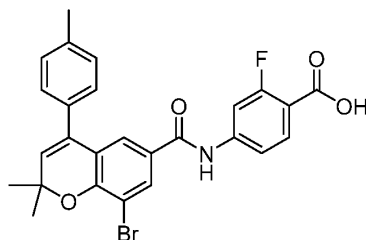
AGN 194301
