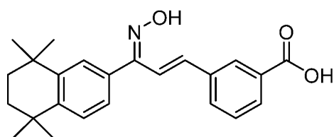
AGN 204647
