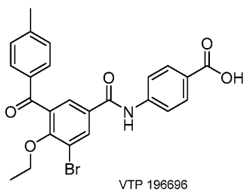
VTP 196696
