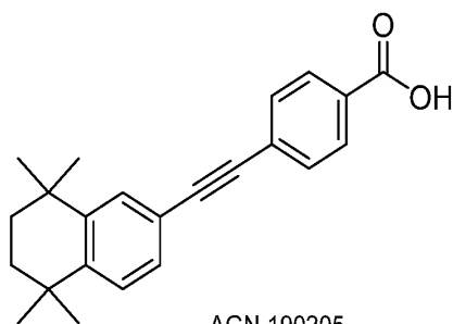
AGN 190205
