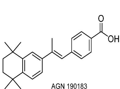
AGN 190183
