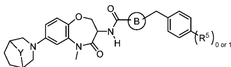
Formula VA
