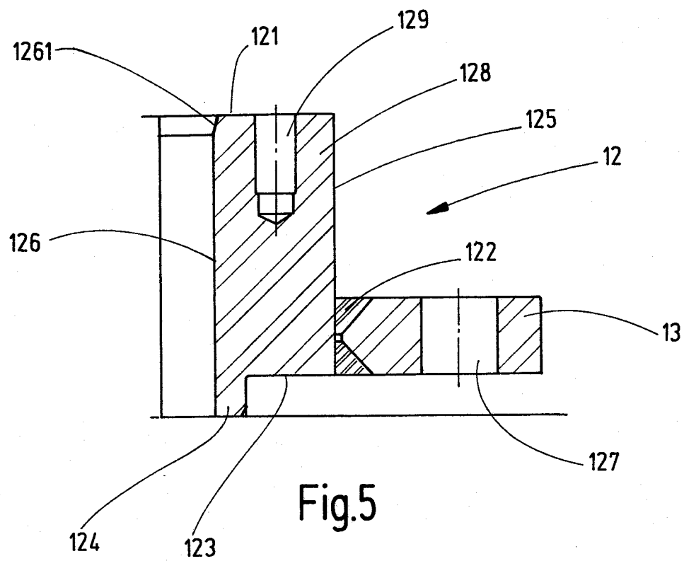
Schnitt B - B
